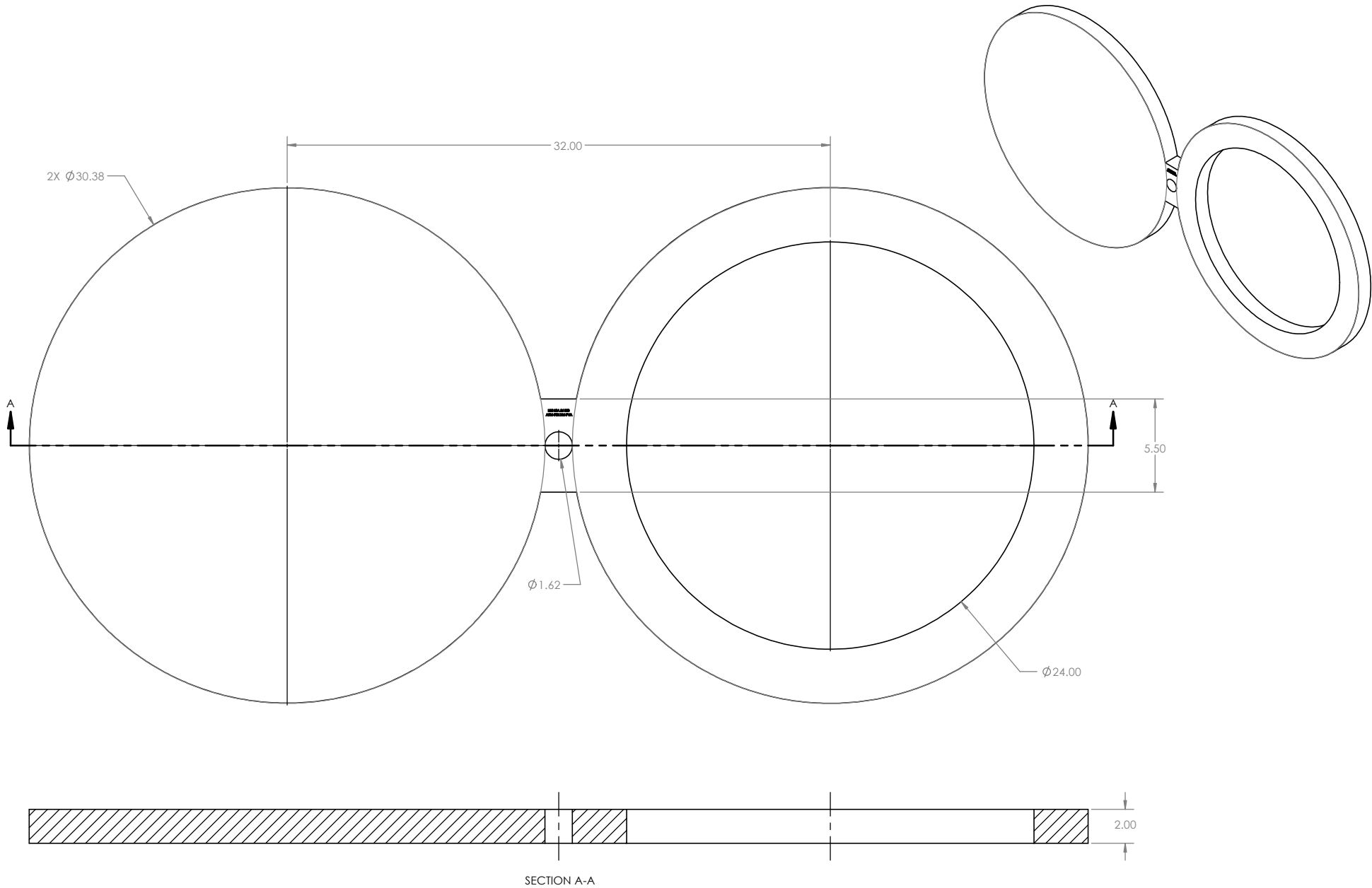
SECTION A-A
